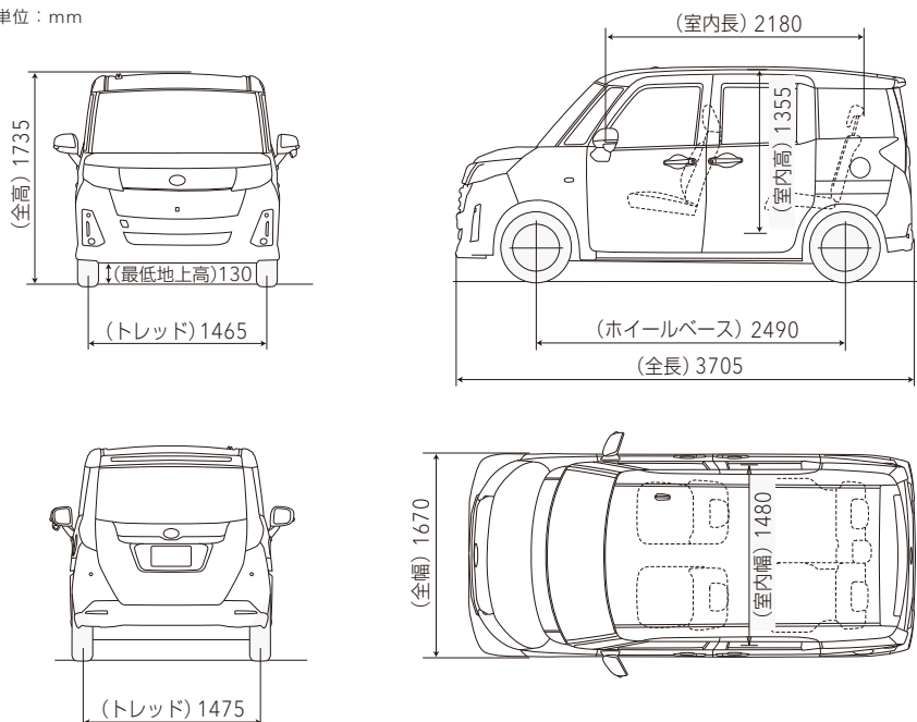
4面図(2WD) 単位: mm
