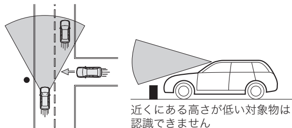
ステレオカメラ視野範囲イメージ
