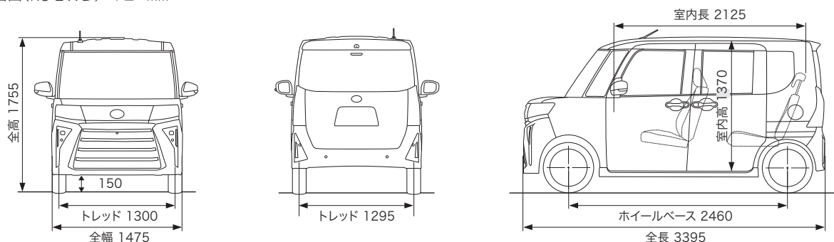
3面図(RS 2WD) 単位：mm
