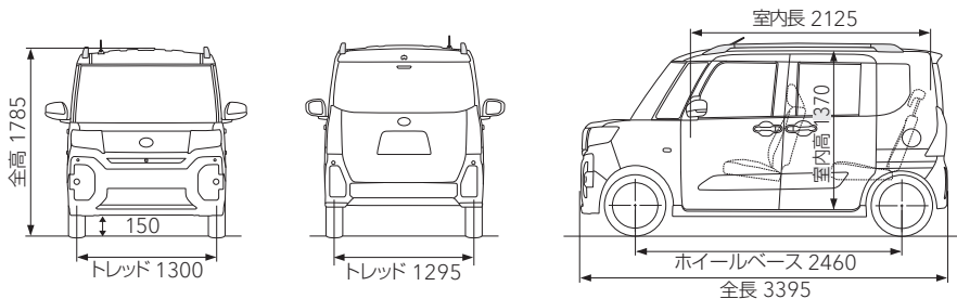
3面図(TRY 2WD) 単位:mm
